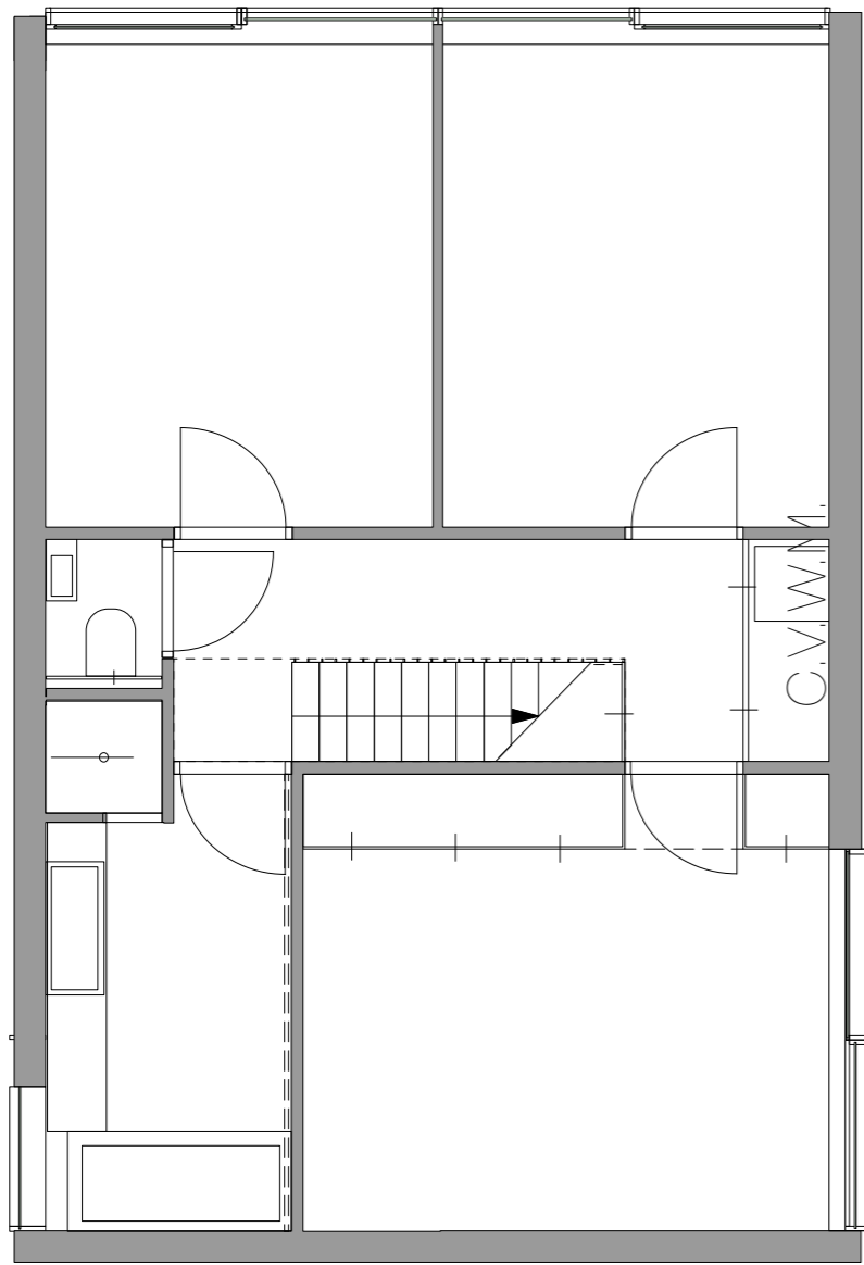
Slaapverdieping
